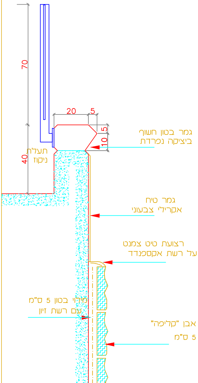
פרט חתך אנכי בקיר בחציבה
