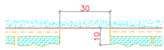
פרט חתך אופקי במרזב אנכי בקיר בחציבה
