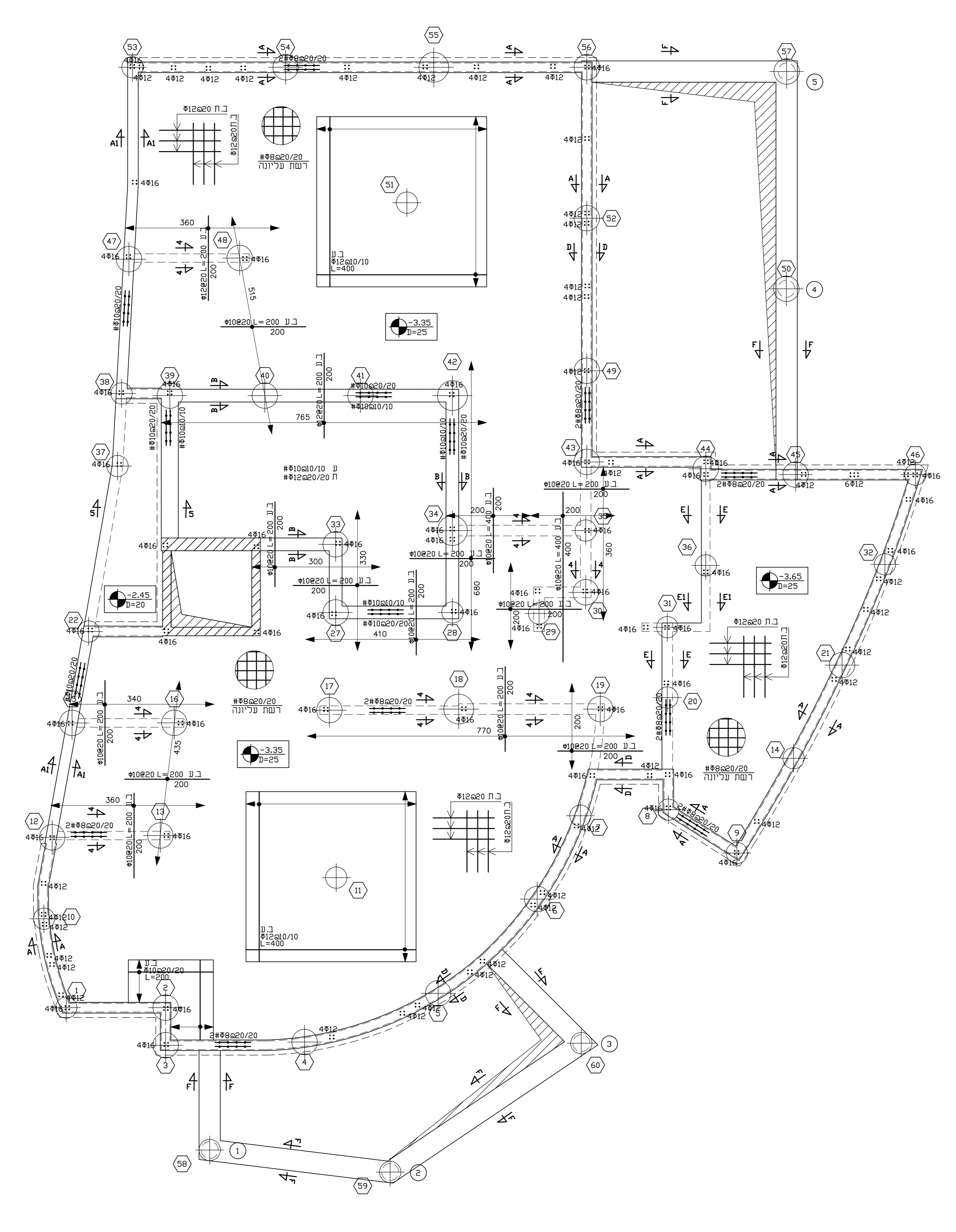
תכנית ברזל
