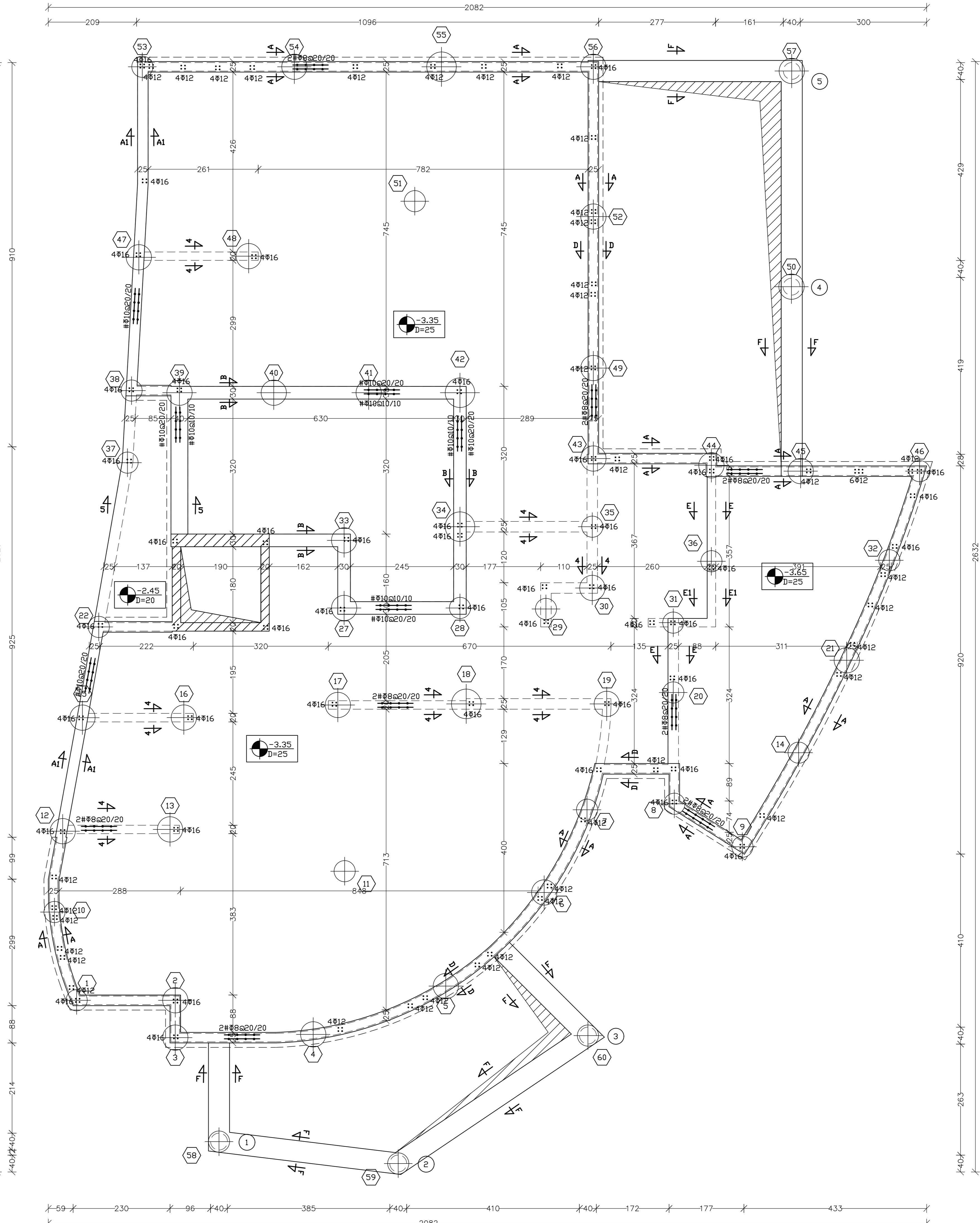
תכנית מידות
