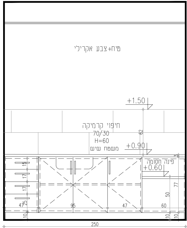
פריסה 1 קנ"מ: 1:25
