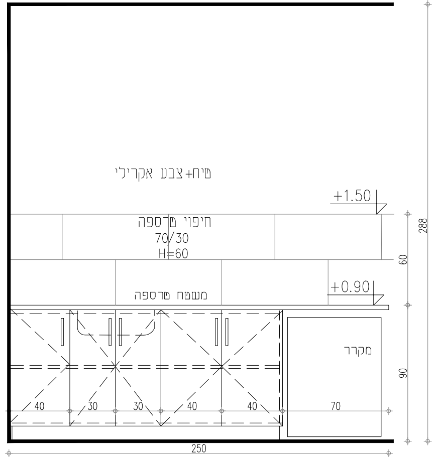
פריסה קנ"מ: 1:25
