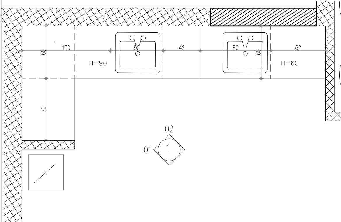
תכנית קנ"מ: 1:25
