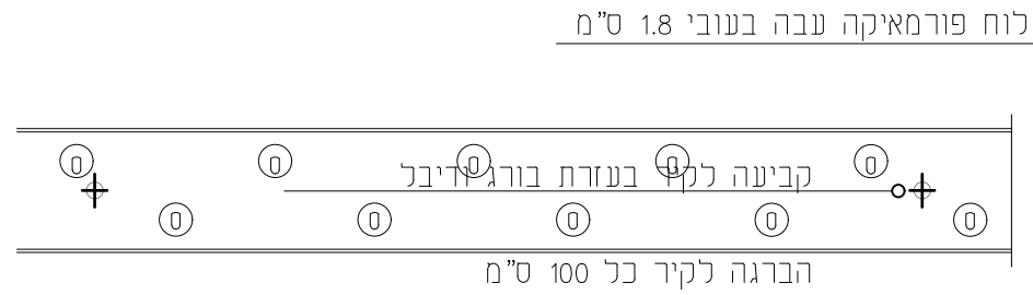
חזית וחתך קנ"מ 1:10
