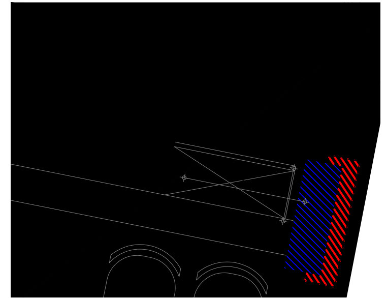
תוכנית ארון קנ"מ 1:25
