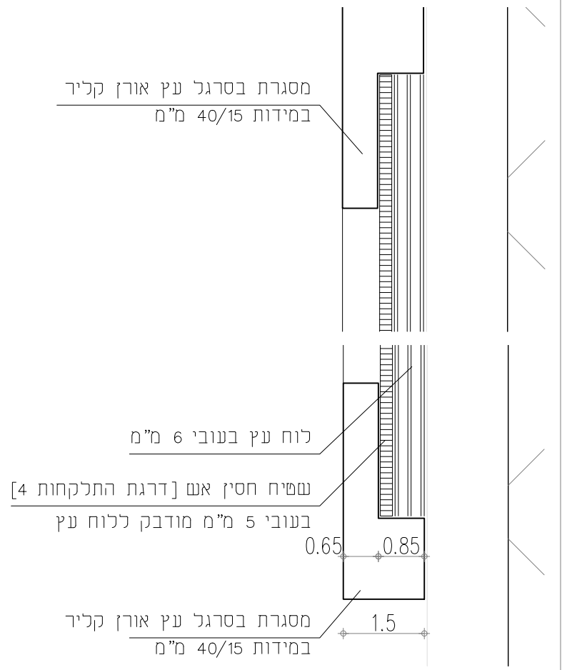
חתך לוח נעיצה קנ"מ 1:1
