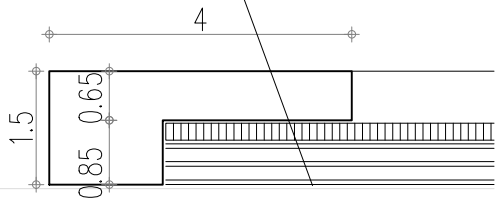
לוח עץ בעובי 6 מ"מ שפיח חסין אש [דרגת התלקחות 4] בעובי 5 מ"מ מודבק ללוח עץ
