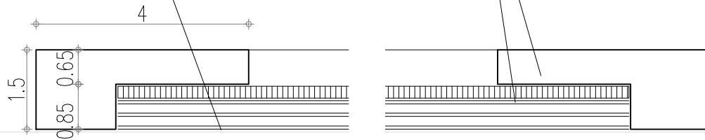
לוח עץ בעובי 6 מ"מ שטיח חסין אש [דרגת התלקחות 4] בעובי 5 מ"מ מודבק ללוח עץ
