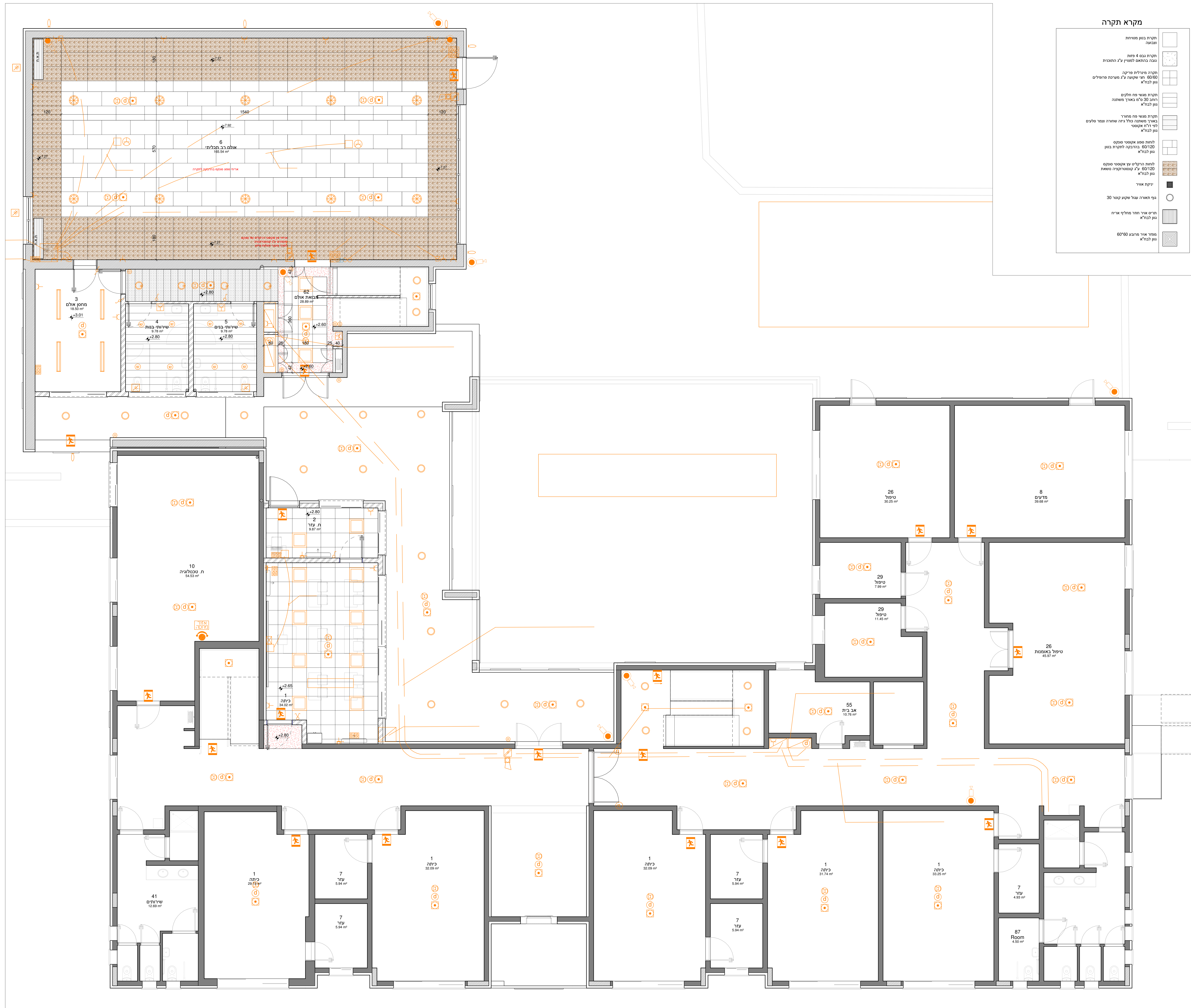
תקרות קומה א 1:50
