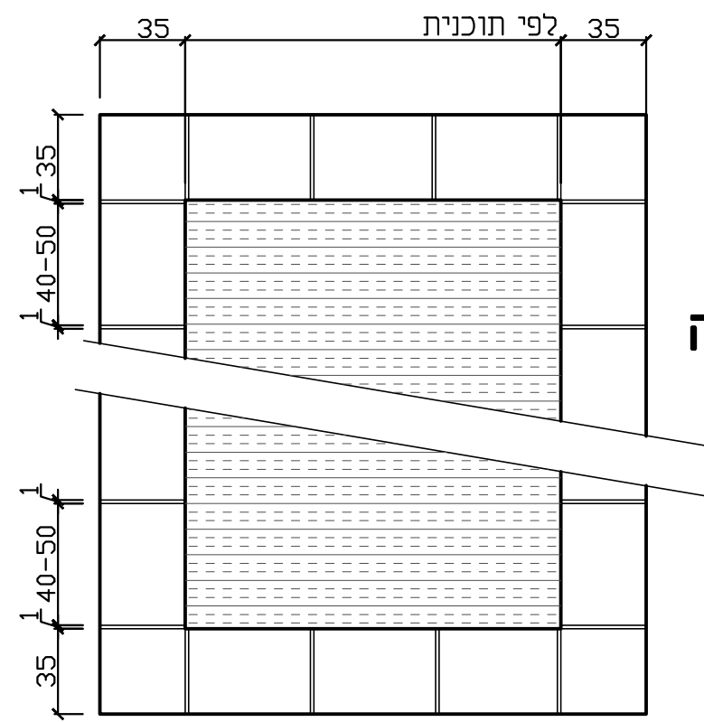
תנוחה 1:20
