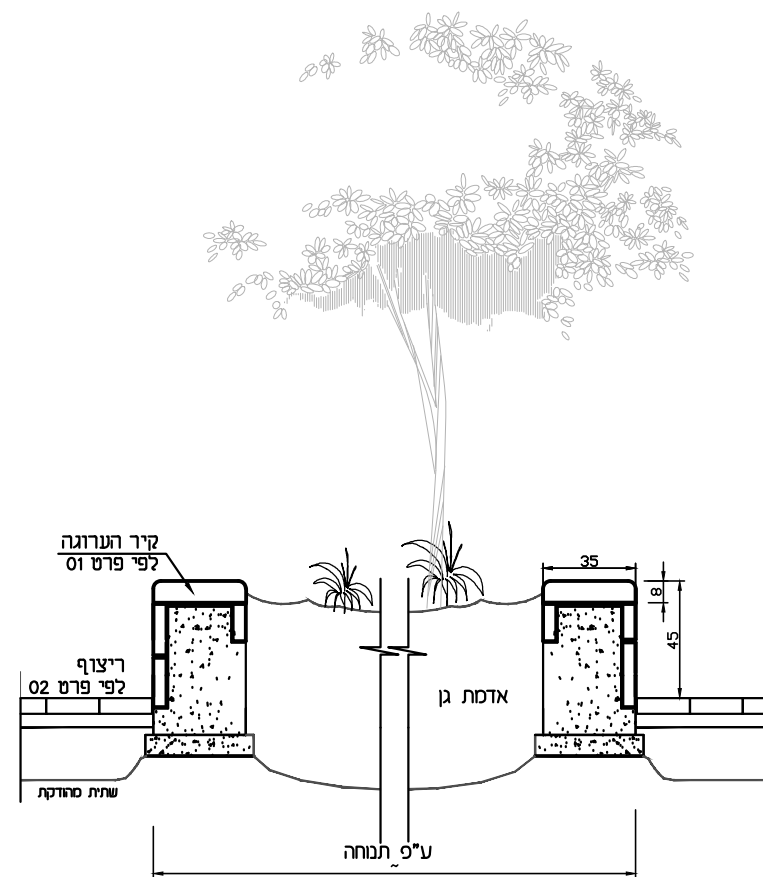
חתך 1:20
