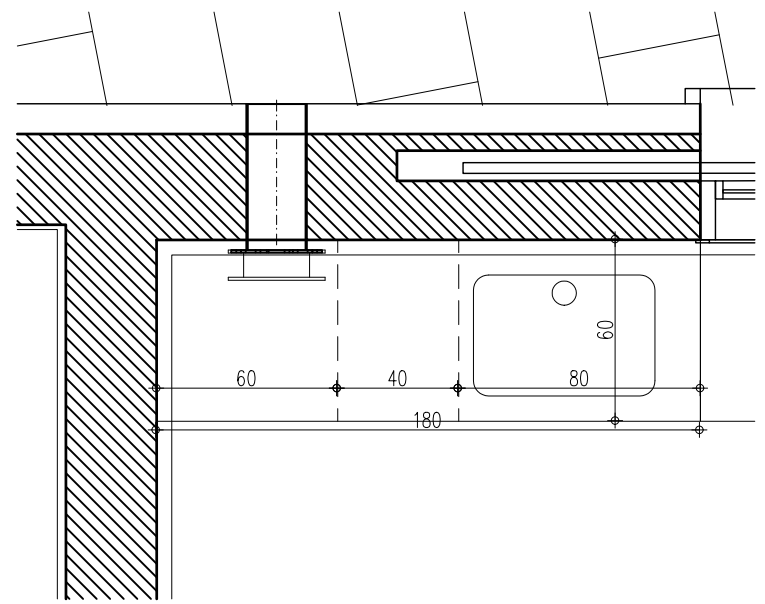
תכנית קנ"מ: 1:25
