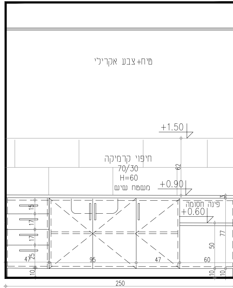
פריסה 1 קנ"מ: 1:25
