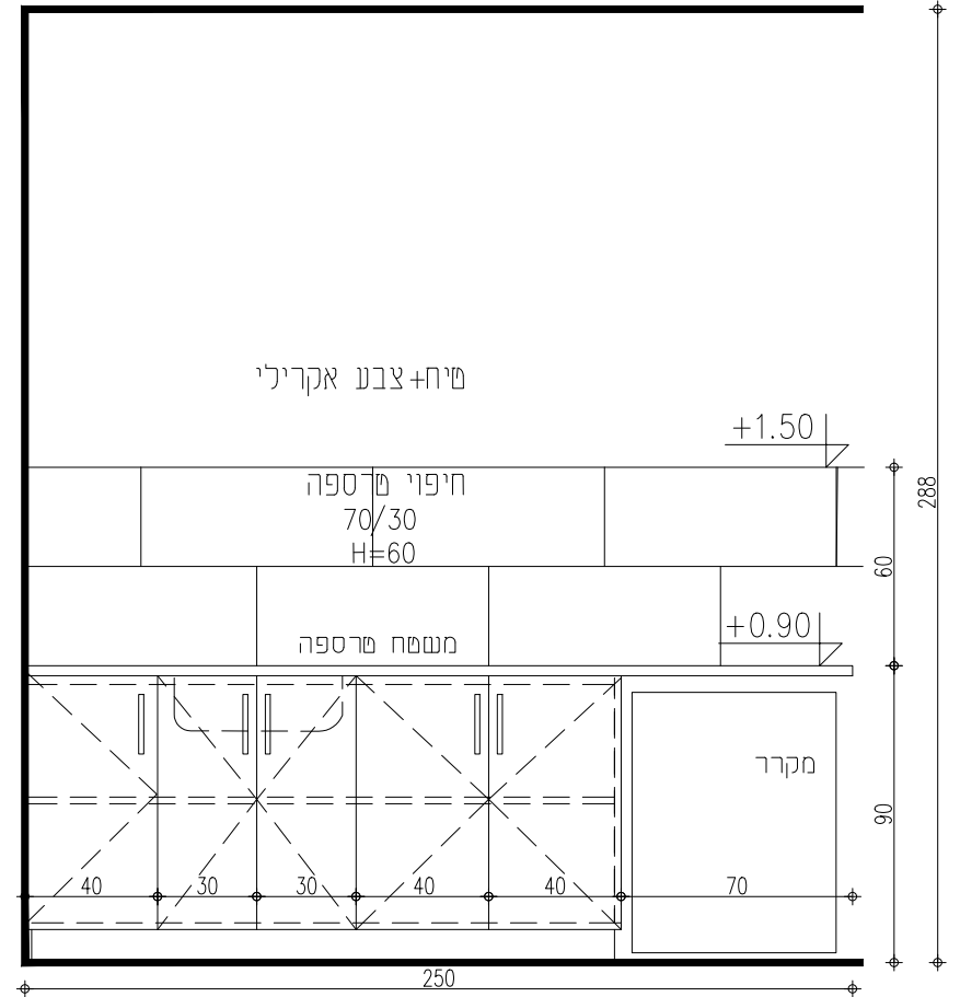
פריסה קנ"מ: 1:25
