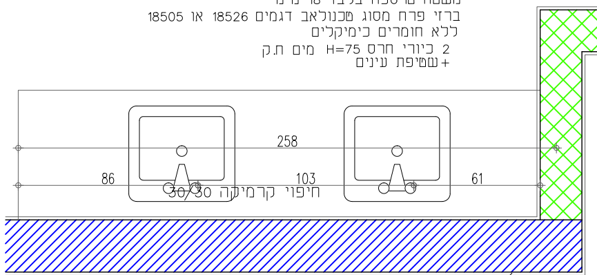
תוכנית ארון קנ"מ 1:25
