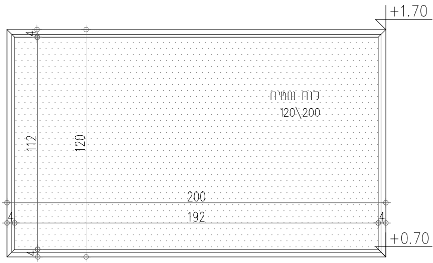
חזית קנ"מ 1:20
