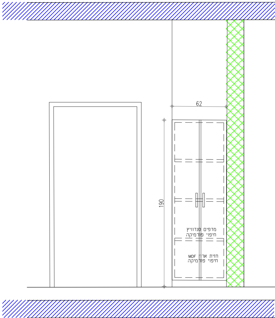
חזית ארון 1:25 מ קנ"מ
