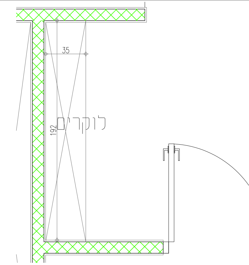
תוכנית ארון קנ"מ 1:50
