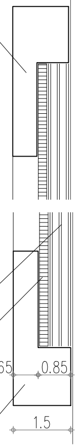
חתך לוח נעיצה קנ"מ 1:1
